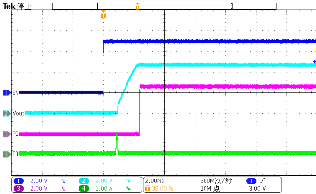
Figure 44. Enable (Iload=10mA)
