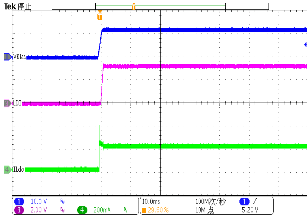
Figure 29. LDO Power up (Ildo=200mA)
