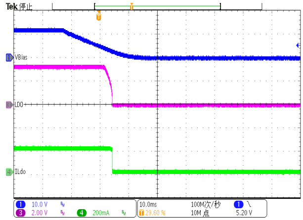
Figure 30. LDO Power down (Ildo=200mA)
